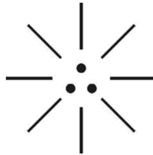
(ATOM)
